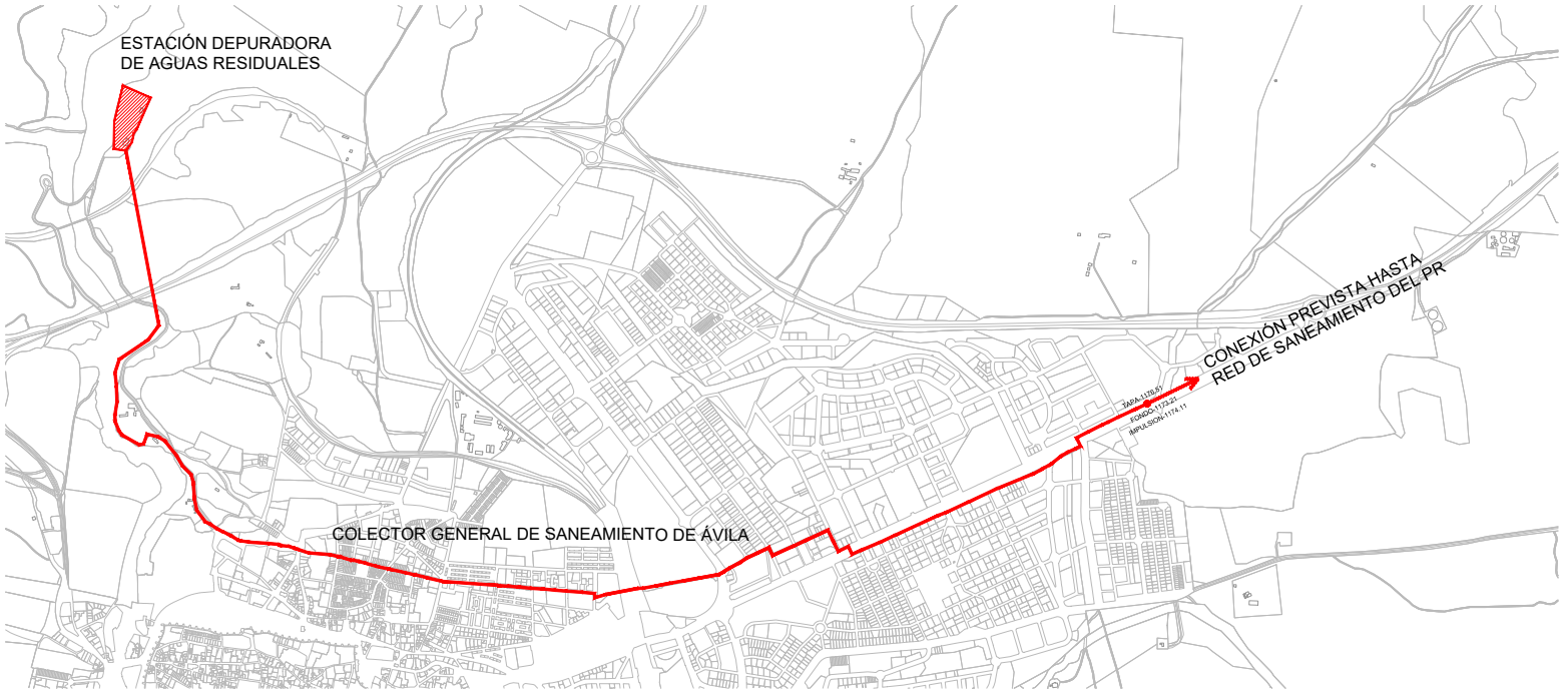
CONEXIÓN DE LA RED DE SANEAMIENTO DEL PR CON EDAR DE ÁVILA. E:1/30.000
